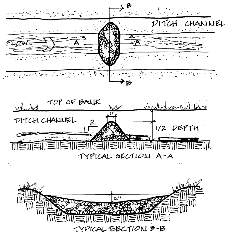
Stone Dike
